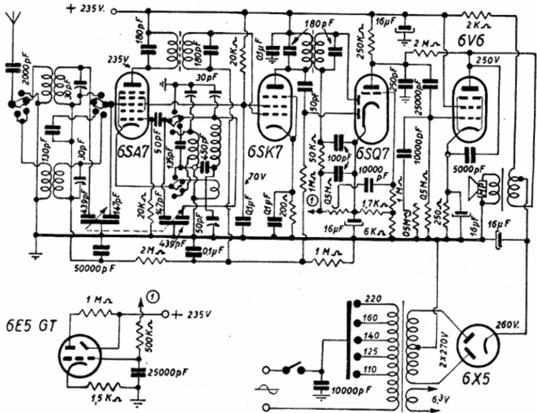
WATT RADIO - Mod. 50 e W/50 ARGO - Medie e due corte. Media frequenza a 470 kc. Finale: placca 250 V, schermo 224 V, griglia 11 V. Massima tensione anodica 260 V. Conv. e ampl. MF: placche 235 V, schermi 70 V.
